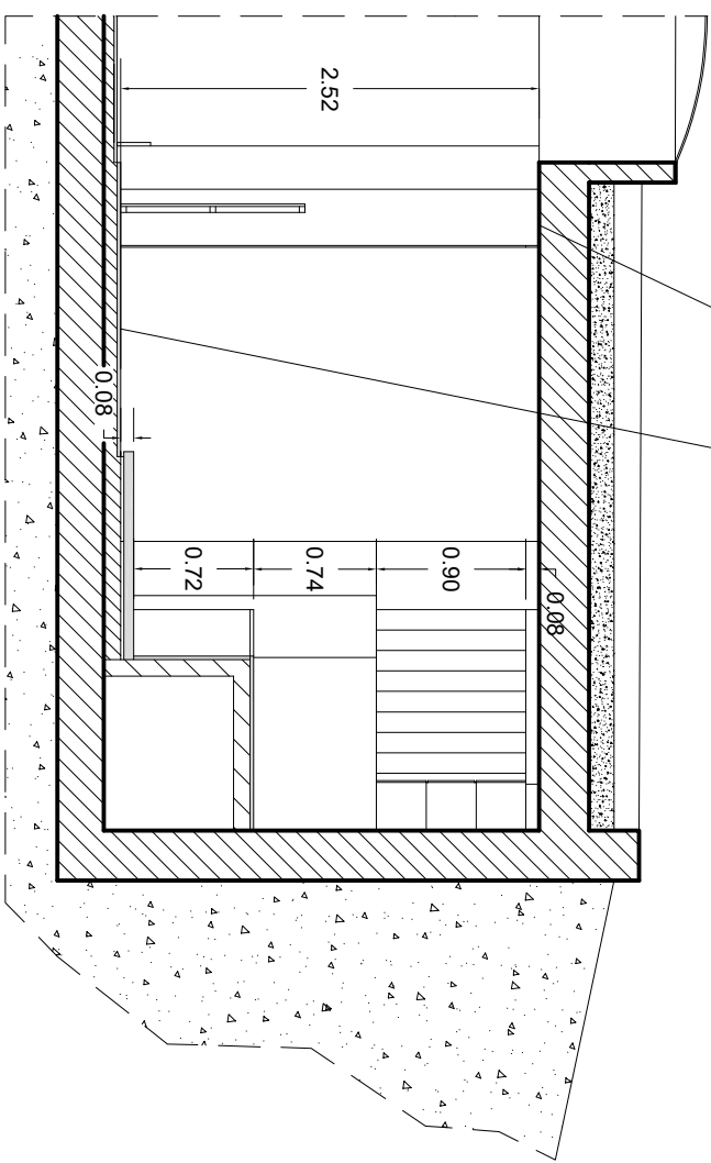
sezione A-A
